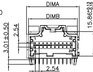
LAYOUT FOR 16&20CKT HEADERS 20 CKT.A Type SHOWN
