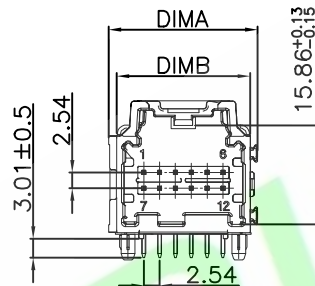
LAYOUT FOR 8&12CKT HEADERS 12CKT.A Type SHOWN
