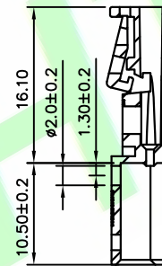
剖面 A-A
