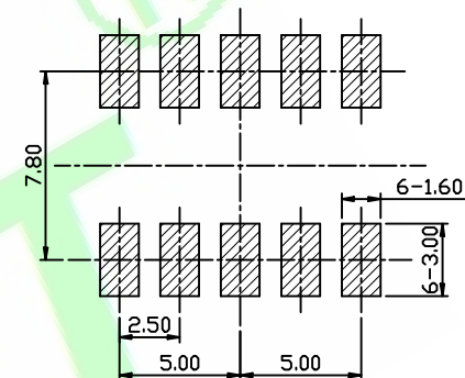
Tolerance: \pm 0.05\text{mm}
