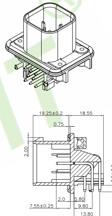
SEC A-A
