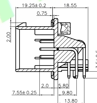
SEC A-A
