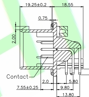
SEC A-A
