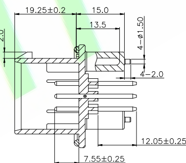
SEC A-A
