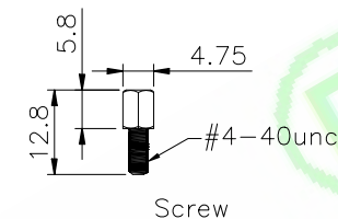
A:Screw length
