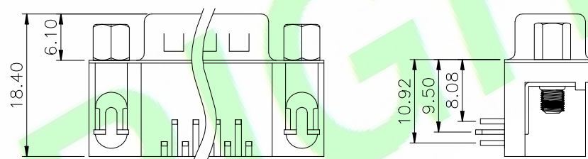
B:Screw length
