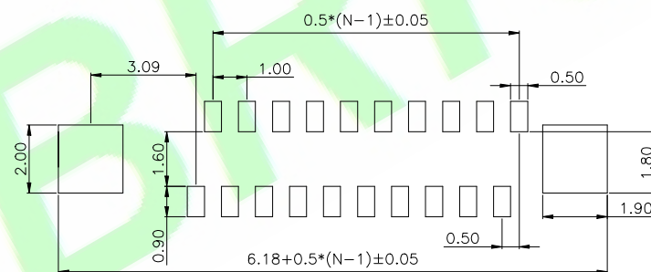
P.C.B Layout
