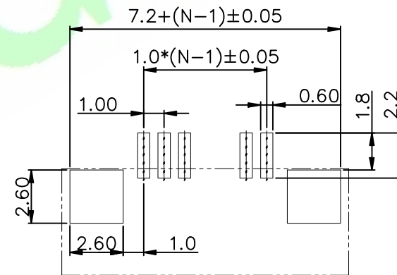
P.C.B Layout recommend
