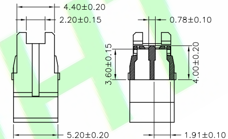
SEC:A-A
