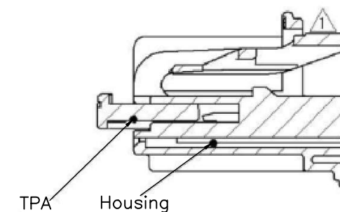
SEC. A-A
