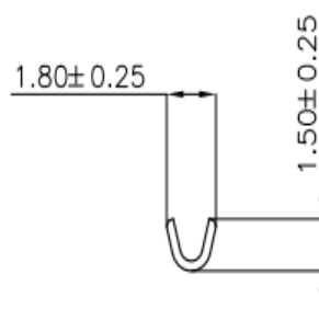
SEC:B-B
